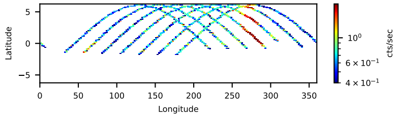
60160255002: 3 to 120 keV
