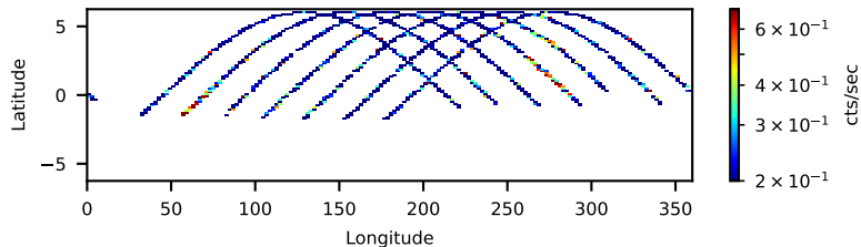
60160255002: 3 to 10 keV
