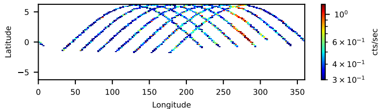
60160255002: 30 to 120 keV
