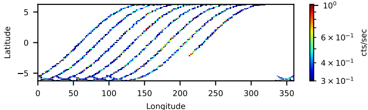
60160232002: 30 to 120 keV
