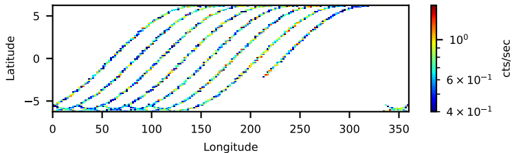
60160232002: 3 to 120 keV
