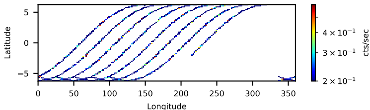
60160232002: 3 to 10 keV
