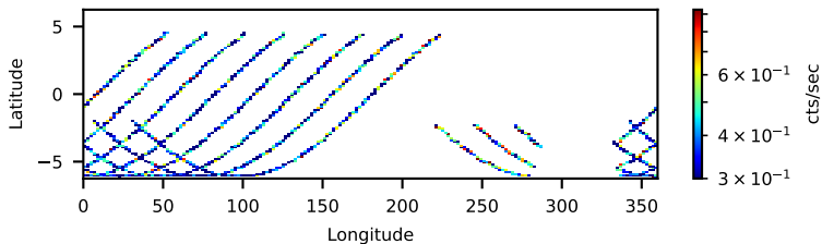
60160181002: 30 to 120 keV
