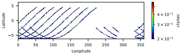
60160181002: 3 to 10 keV
