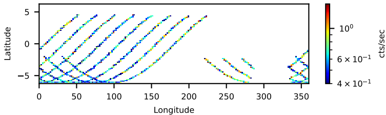
60160181002: 3 to 120 keV
