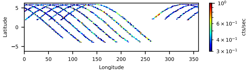
60160148002: 30 to 120 keV
