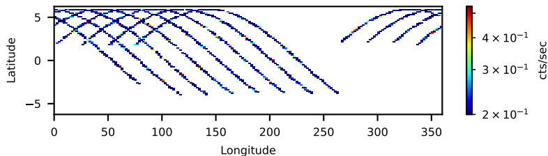
60160148002: 3 to 10 keV
