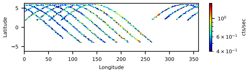
60160148002: 3 to 120 keV
