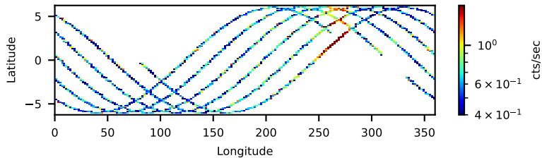
60160141002: 3 to 120 keV
