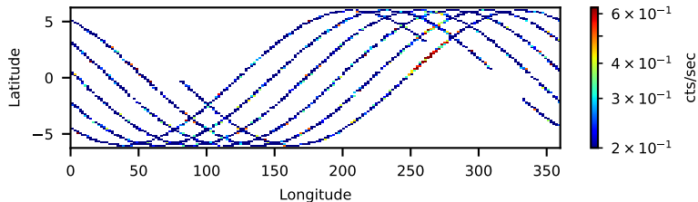
60160141002: 3 to 10 keV
