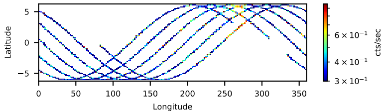
60160141002: 30 to 120 keV
