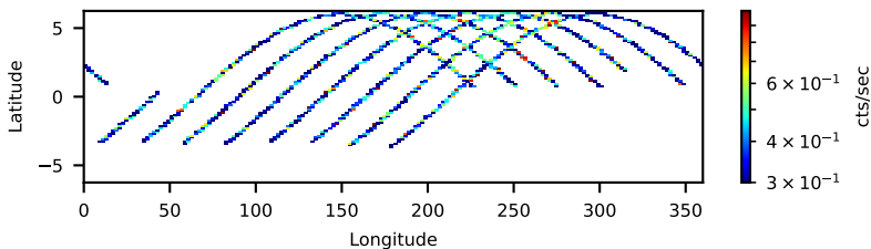
60160133002: 30 to 120 keV
