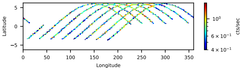
60160133002: 3 to 120 keV
