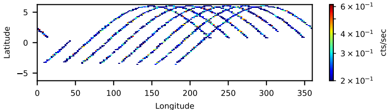
60160133002: 3 to 10 keV
