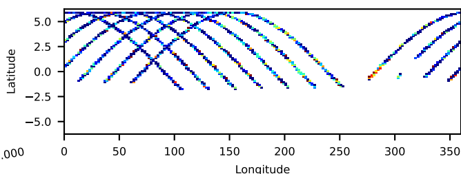
60160119002: 30 to 120 keV
