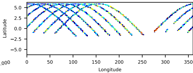
60160119002: 3 to 10 keV
