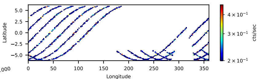
60160115002: 3 to 10 keV
