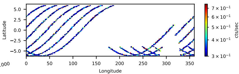
60160115002: 30 to 120 keV
