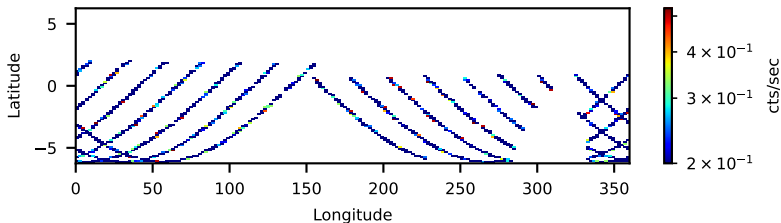
60160088002: 3 to 10 keV
