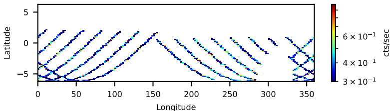
60160088002: 30 to 120 keV
