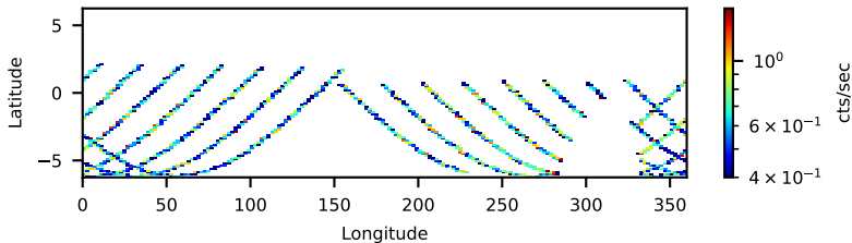
60160088002: 3 to 120 keV
