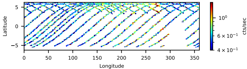
60111035001: 3 to 120 keV
