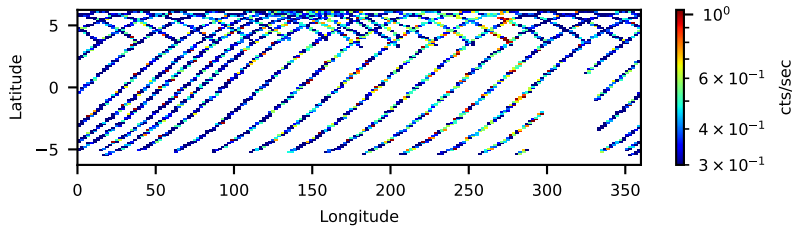
60111035001: 30 to 120 keV
