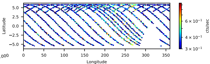
60111012001: 30 to 120 keV
