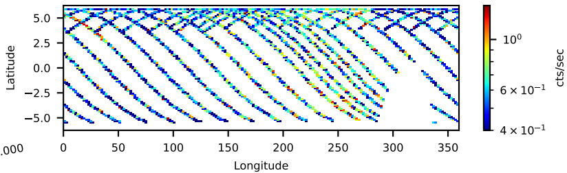
60111012001: 3 to 10 keV
