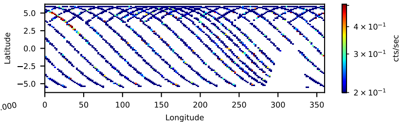
60111012001: 30 to 120 keV
