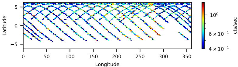
60111010001: 3 to 120 keV
