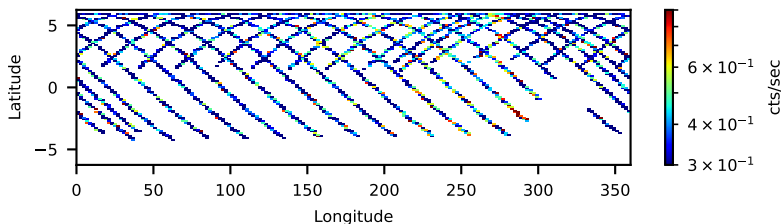
60111010001: 30 to 120 keV
