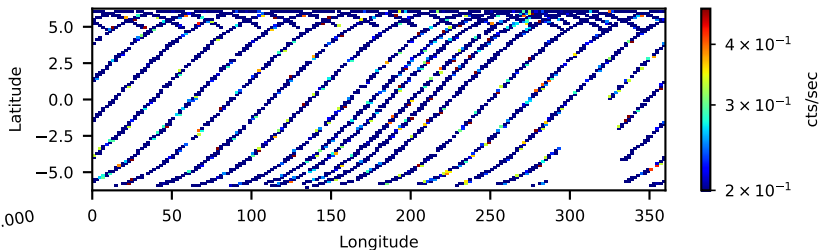
60111003002: 30 to 120 keV
