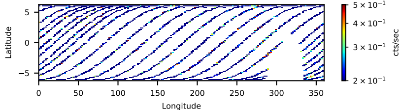
60111002002: 3 to 10 keV
