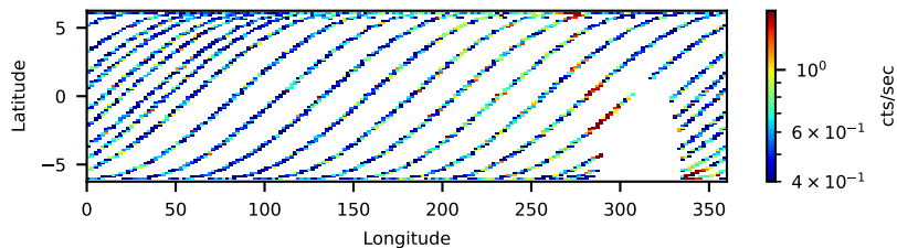
60111002002: 3 to 120 keV
