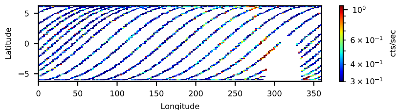
60111002002: 30 to 120 keV
