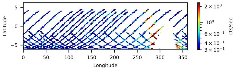
60101102002: 30 to 120 keV
