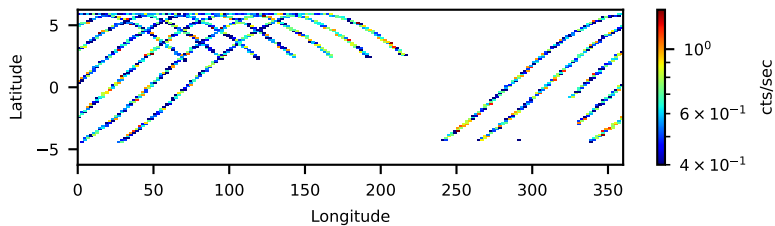
60101069002: 3 to 120 keV
