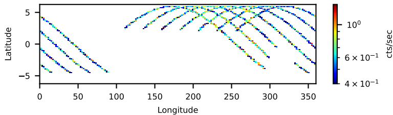
60061340002: 3 to 120 keV
