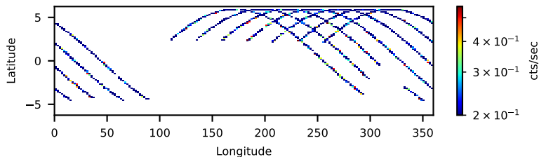
60061340002: 3 to 10 keV
