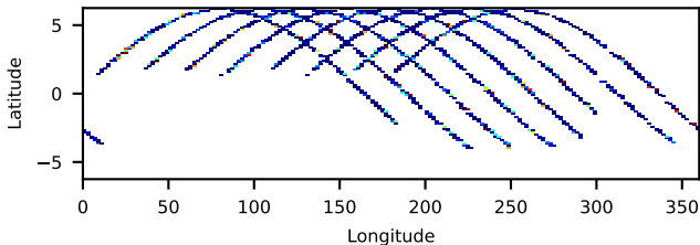
60061250002: 3 to 10 keV
