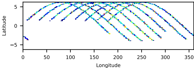
60061250002: 3 to 120 keV
