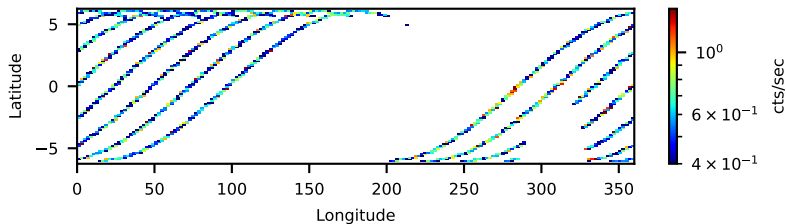
60061220002: 3 to 120 keV
