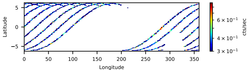
60061220002: 30 to 120 keV
