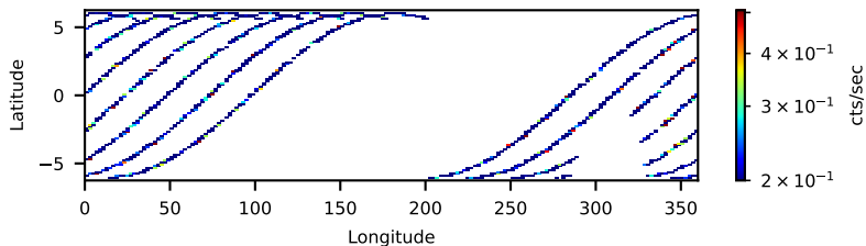
60061220002: 3 to 10 keV
