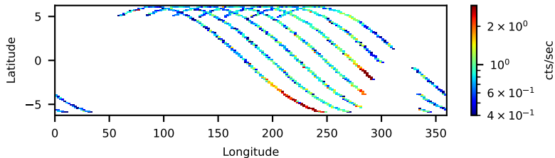
60061218002: 3 to 120 keV
