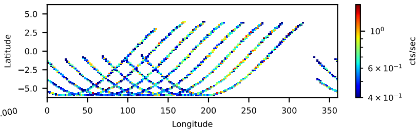
60061217006: 3 to 10 keV
