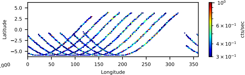
60061217006: 30 to 120 keV
