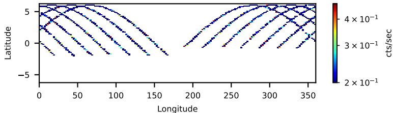
60061069002: 3 to 10 keV
