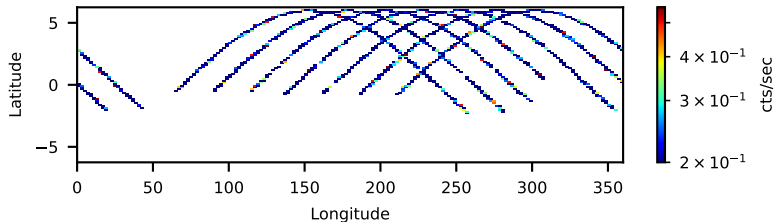
60061056002: 3 to 10 keV
