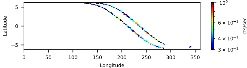
60061044002: 30 to 120 keV
