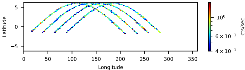
60061039004: 3 to 120 keV
