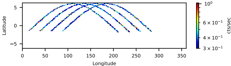
60061039004: 30 to 120 keV
