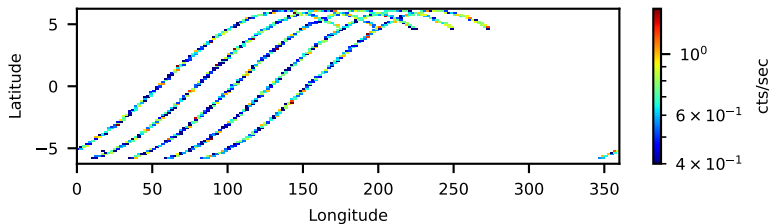
60061018002: 3 to 120 keV
