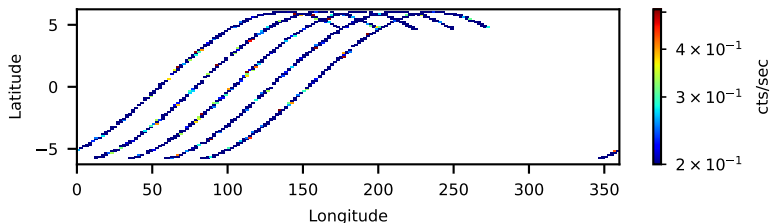
60061018002: 3 to 10 keV
