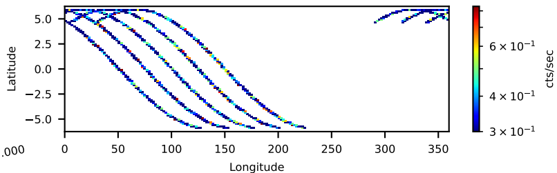
60061012002: 30 to 120 keV
