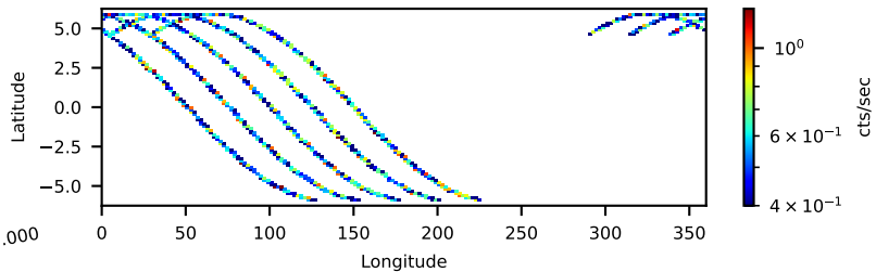
60061012002: 3 to 10 keV
