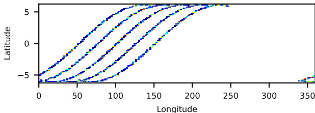
60061007002: 30 to 120 keV
