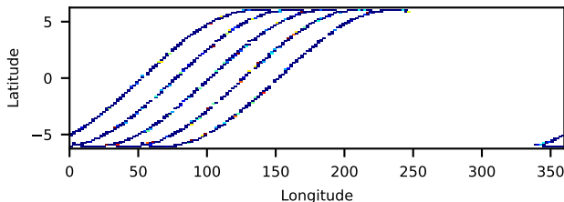
60061007002: 3 to 10 keV
