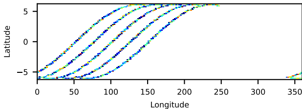
60061007002: 3 to 120 keV
