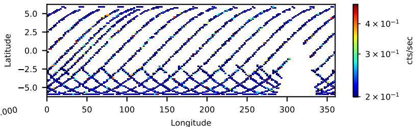
60023006005: 30 to 120 keV
