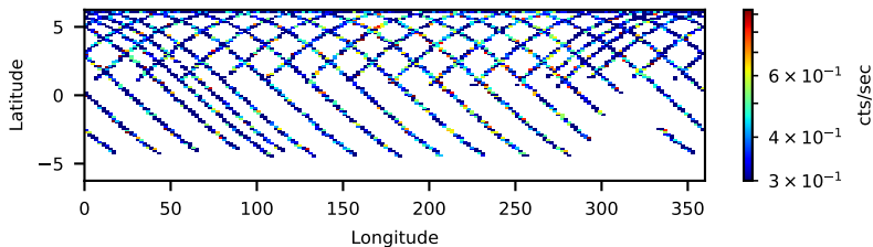
60023005004: 30 to 120 keV
