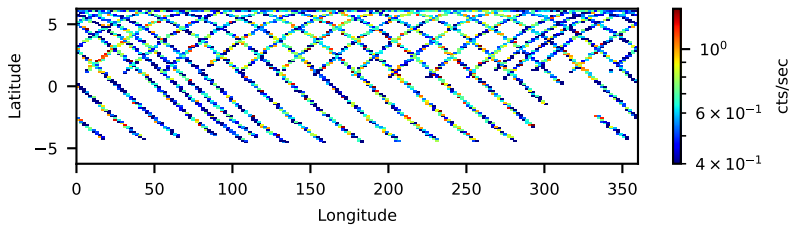
60023005004: 3 to 120 keV
