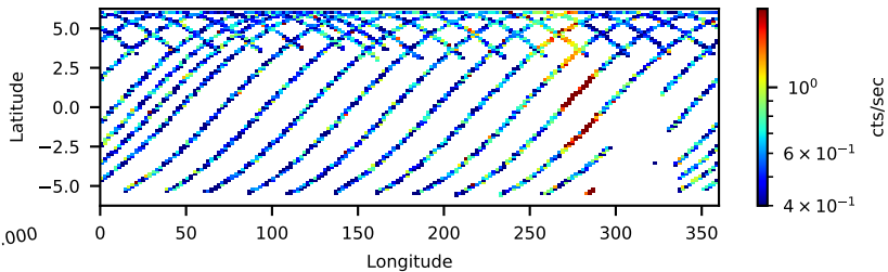
60022015003: 3 to 10 keV
