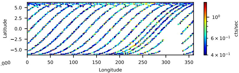
60022010001: 3 to 10 keV
