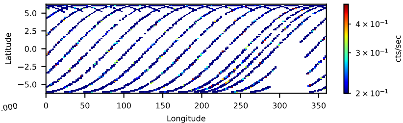
60022010001: 30 to 120 keV
