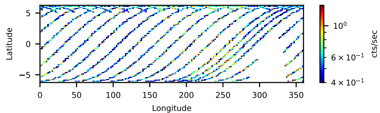
60022010001: 3 to 120 keV
