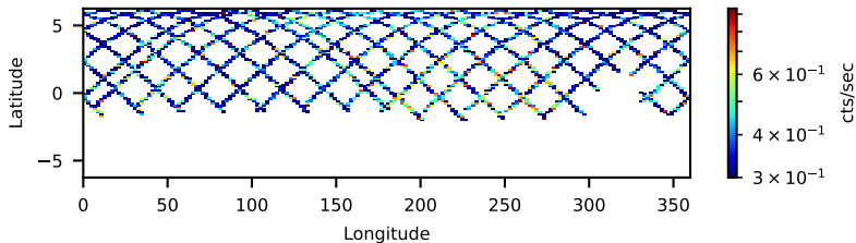
60022009003: 30 to 120 keV
