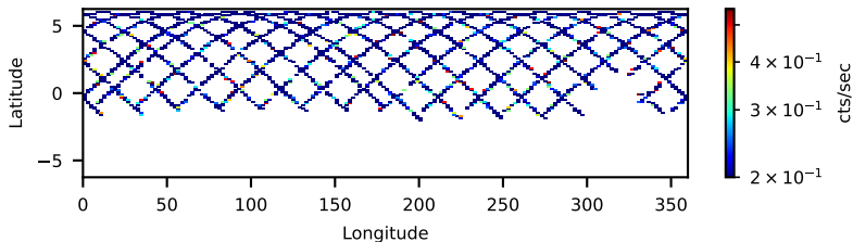
60022009003: 3 to 10 keV
