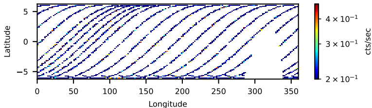
60022007002: 3 to 10 keV
