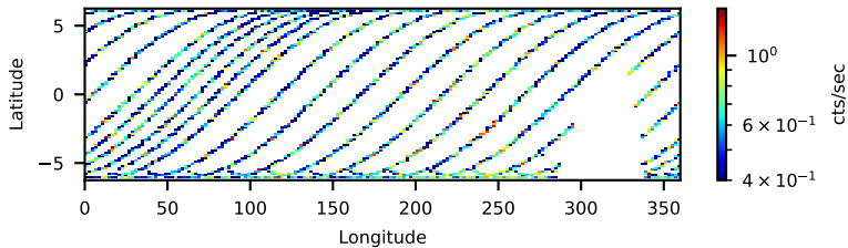
60022007002: 3 to 120 keV
