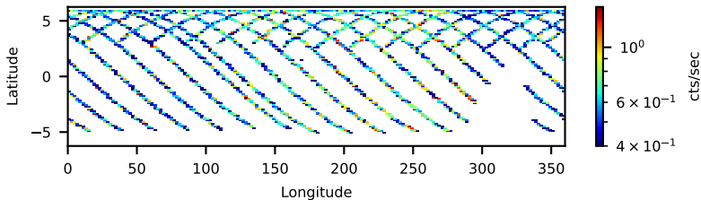
60022004002: 3 to 120 keV
