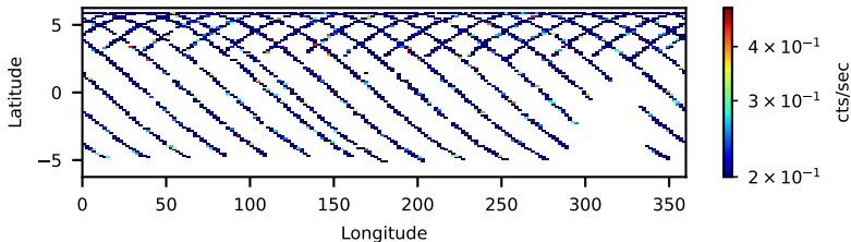
60022004002: 3 to 10 keV
