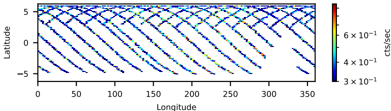
60022004002: 30 to 120 keV
