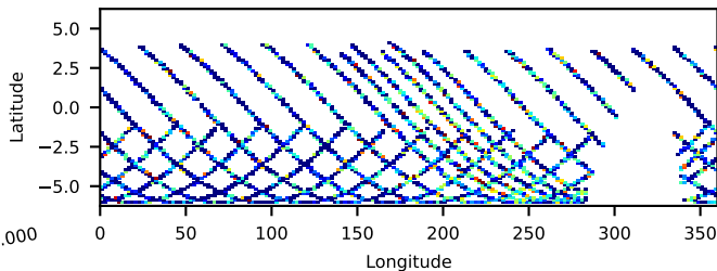
60022001002: 30 to 120 keV
