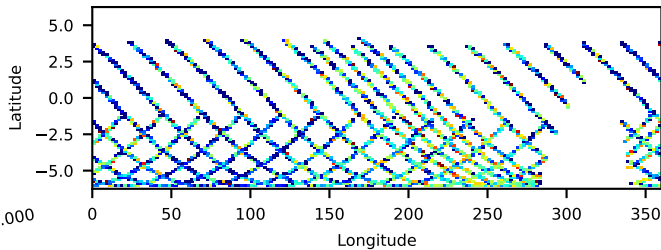
60022001002: 3 to 10 keV
