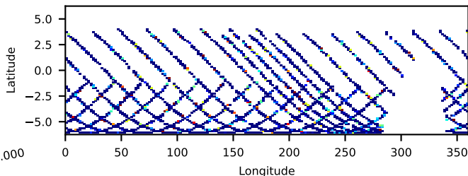
60022001002: 30 to 120 keV
