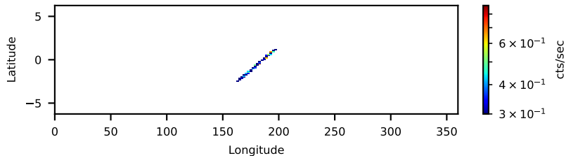
60002049009: 30 to 120 keV
