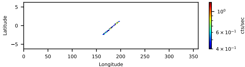
60002049009: 3 to 120 keV
