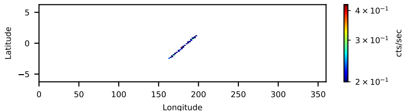
60002049009: 3 to 10 keV
