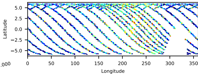
60002033002: 3 to 10 keV
