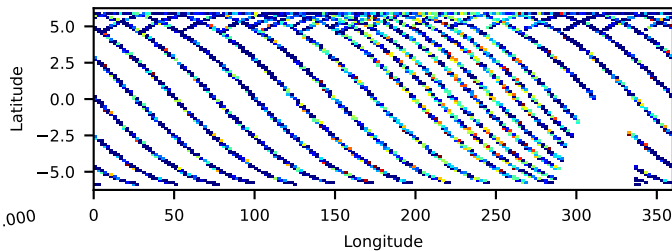
60002033002: 30 to 120 keV
