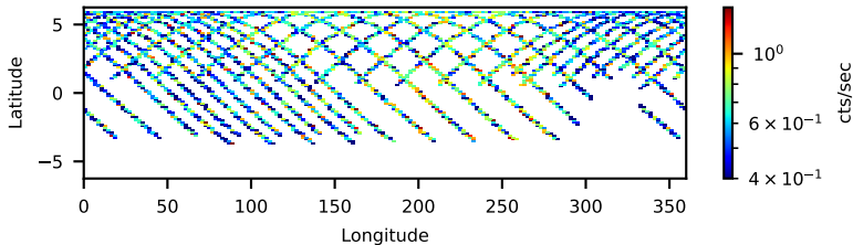
60002030002: 3 to 120 keV
