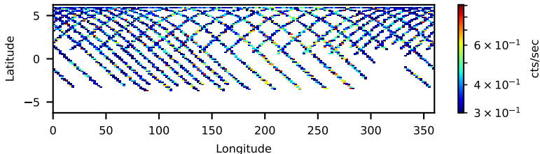
60002030002: 30 to 120 keV
