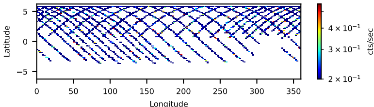
60002030002: 3 to 10 keV
