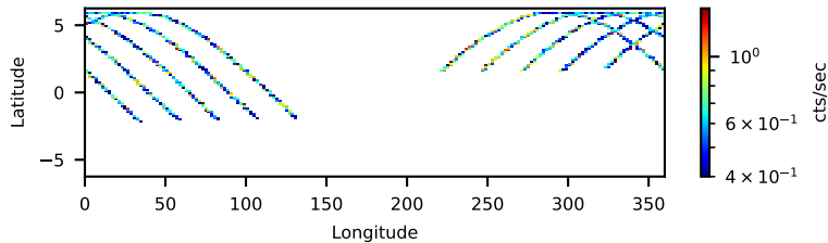
60002022004: 3 to 120 keV
