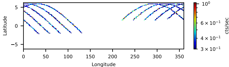
60002022004: 30 to 120 keV
