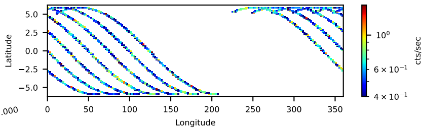
60001161002: 3 to 10 keV
