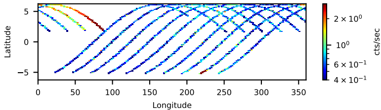
60001157002: 3 to 120 keV
