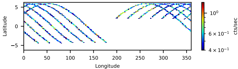
60001144002: 3 to 120 keV
