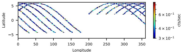
60001144002: 30 to 120 keV
