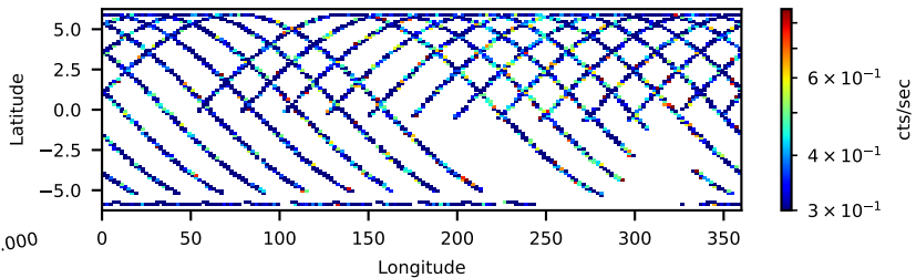
60001130002: 30 to 120 keV
