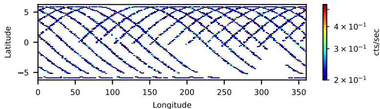
60001130002: 3 to 10 keV
