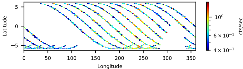
60001112002: 3 to 120 keV
