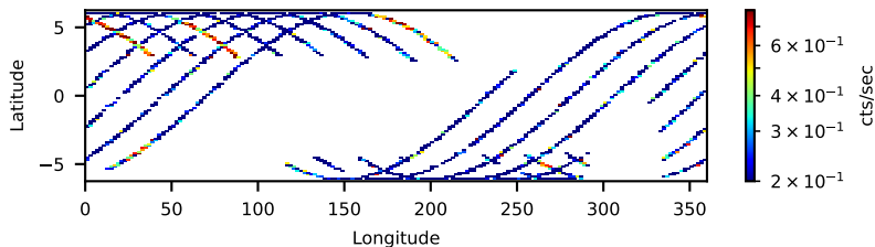
60001098002: 3 to 10 keV
