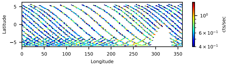
60001044004: 3 to 120 keV
