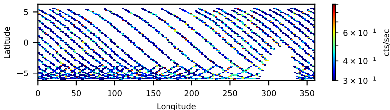
60001044004: 30 to 120 keV
