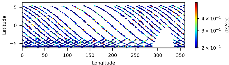
60001044004: 3 to 10 keV
