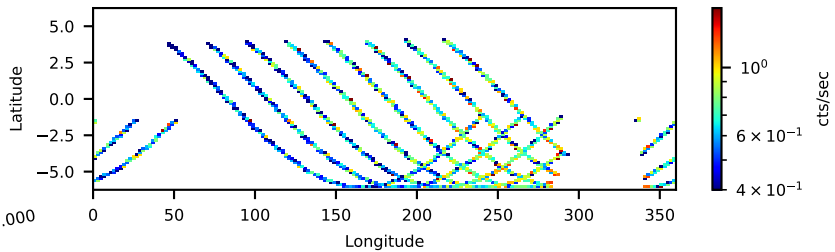
60001041002: 3 to 10 keV
